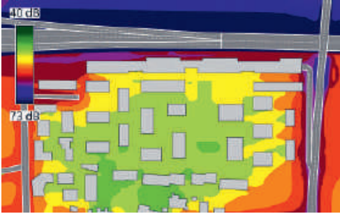
Dans le quartier Eikenott, créé en 2014 à Gland, un parking à étages de 600 places boisé et végétalisé sert de mur antibruit le long de l'autoroute.
